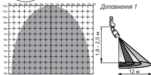
Схема зон охоплення датчика (180°):
